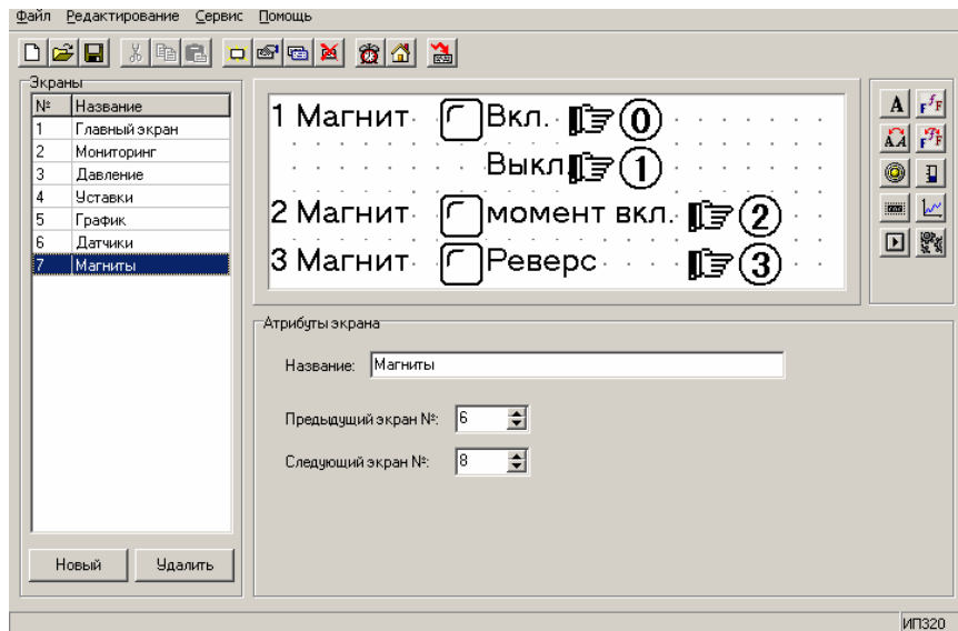
Рис. 7.16. Экран «Магниты»
